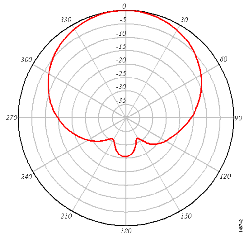
H-Plane Pattern
