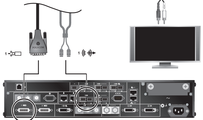
Polycom HDX 9006
